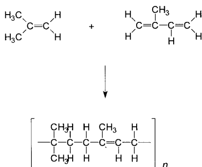
8.7 Butyl rubber.
