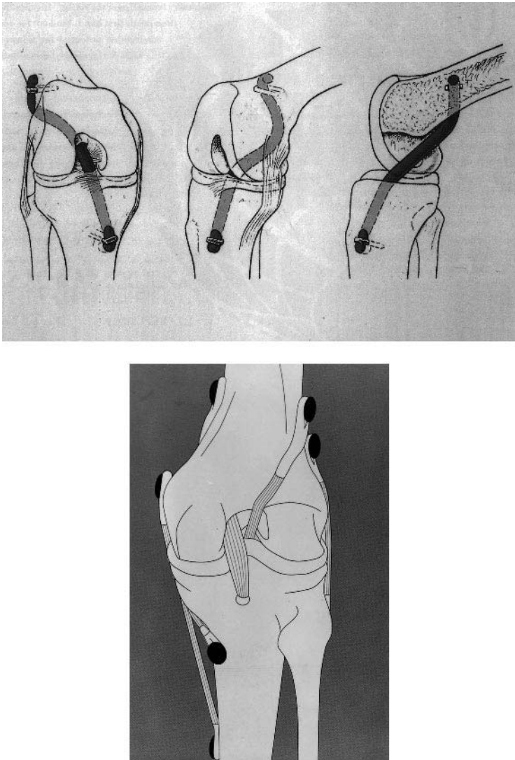
15.6 Anterior cruciate ligament prostheses.
